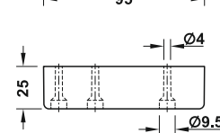
Trojúhelníková k přišroubování
