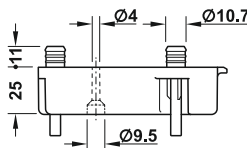
Trojúhelníková k naklepání
