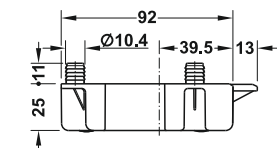
Obdélníkové k nalisování
